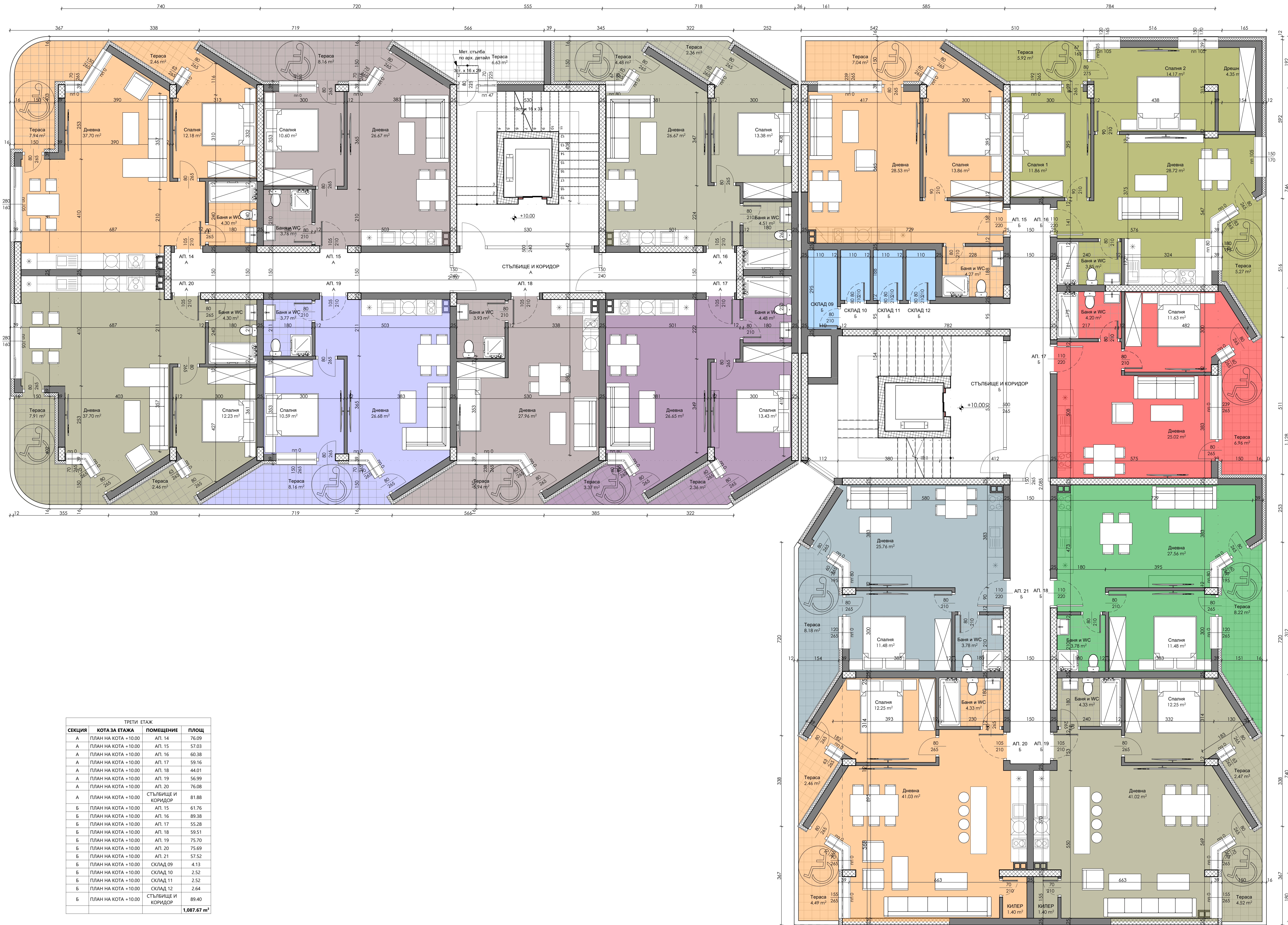
ПЛАН НА КОТА +10.00
